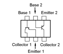
IMZ2 (Z2) (Q1057)
