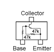
RT1N441U (N3) (Q1042, 1053)
