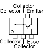
CPH6102 (AB) (Q1029, 1031)
