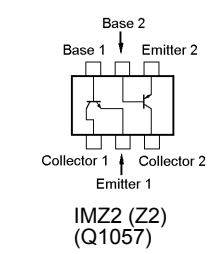
IMZ2 (Z2) (Q1057)
