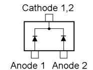
DAN235E (M) (D1014)
