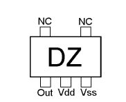
S-80735SN (DZ) (Q1041)
