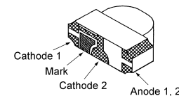
12-22SURSYGC/S530-A2/TR8 (D1026)
