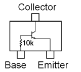
DTC124TE (05) (Q1058)
