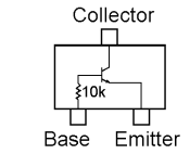
PDTOC114TE (24) (Q1058)
