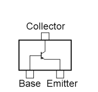
2SA1586Y (SY) (Q1056, 1062)
