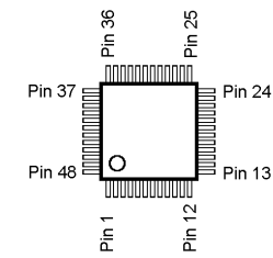
M37516M6 (Q1014)
