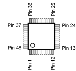
M37516M6 (Q1014)
