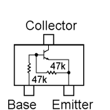
RT1N441U (N3) (Q1042, 1053)
