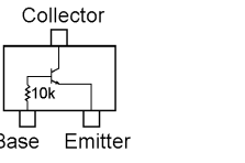
DTC124TE (05) (Q1058)
