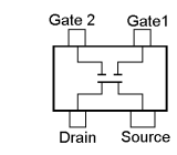
SGM2016AM (MA) (Q1026)
