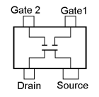
3SK299 (Q1026)
