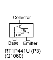
RT1P441U (P3) (Q1060)
