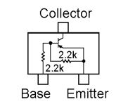
DTB123EK (F12) (Q1036)
