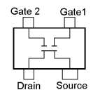
3SK299 (Q1026)
