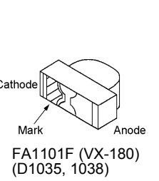
FA1101F (VX-180) (D1035, 1038)
