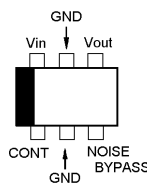
TK11250BMCL (Q1040)
