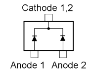
DAN235E (M) (D1014)
