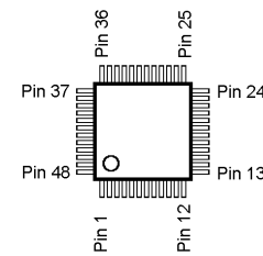
M37516M6 (Q1014)
