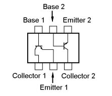
IMZ2 (Z2) (Q1057)
