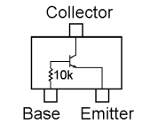
PDTCT114TE (24) (Q1058)
