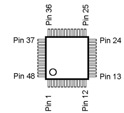
LC75834W (Q1054)
