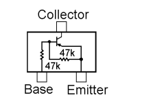
RT1P441U (P3) (Q1060)
